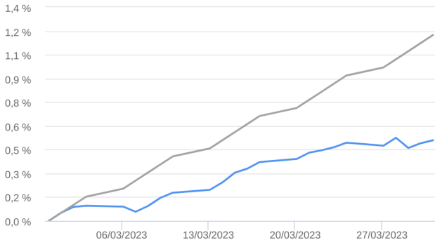
Retorno Acumulado - 01/03/2023 a 31/03/2023 (diária)
