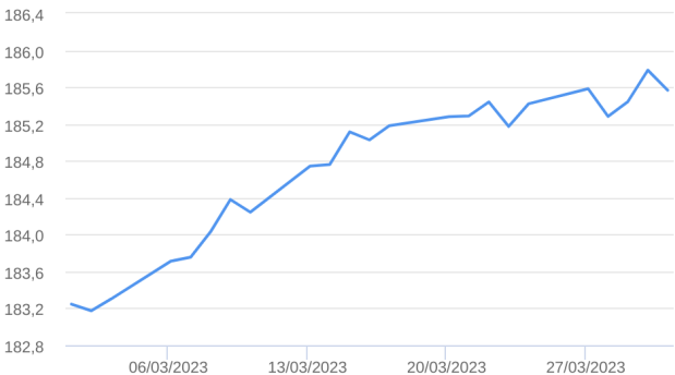
Patrimônio Líquido (R$ Milhões) - 01/03/2023 a 31/03/2023 (diária)
