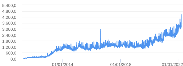
Patrimônio Líquido (R$ Milhões) - 29/04/2011 a 02/03/2022 (diária)
