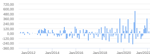
Fluxo Mensal (R$ Milhões) - 29/04/2011 a 02/03/2022 (mensal)
