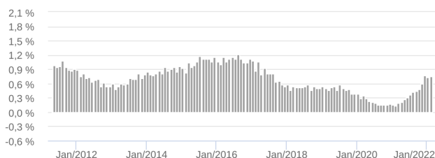
Retorno Mensal - 29/04/2011 a 02/03/2022 (mensal)
