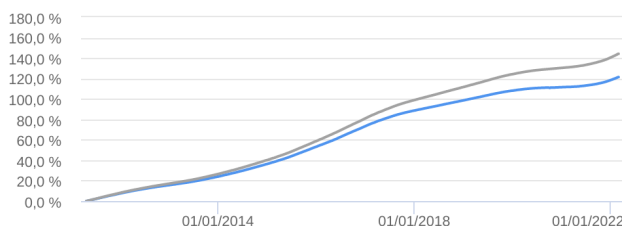
Retorno Acumulado - 29/04/2011 a 02/03/2022 (diária)
