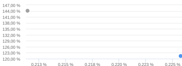
Risco x Retorno - 29/04/2011 a 02/03/2022 (diária)
