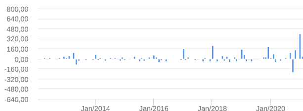
Fluxo Mensal (R$ Milhões) - 17/02/2012 a 20/04/2021 (mensal)
