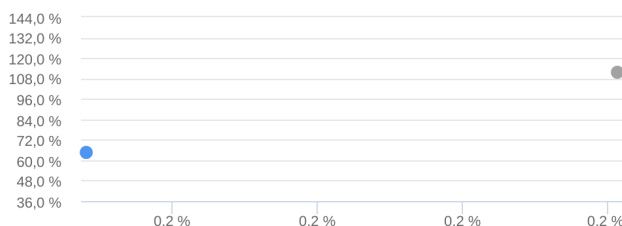
Risco x Retorno - 17/02/2012 a 20/04/2021 (diária)
