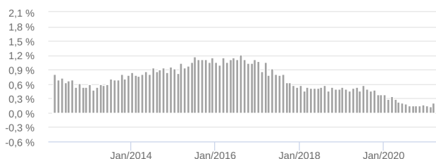
Retorno Mensal - 17/02/2012 a 20/04/2021 (mensal)
