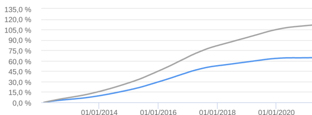
Retorno Acumulado - 17/02/2012 a 20/04/2021 (diária)
