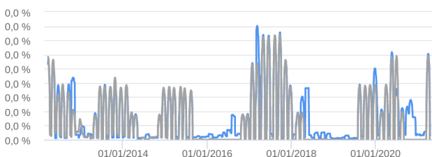
Volatilidade Anualizada - 17/02/2012 a 20/04/2021 (diária)
