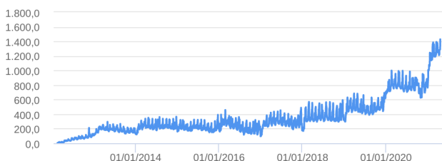
Patrimônio Líquido (R$ Milhões) - 17/02/2012 a 20/04/2021 (diária)
