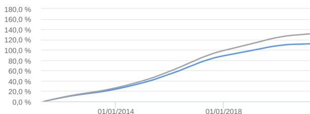
Retorno Acumulado - 29/04/2011 a 22/04/2021 (diária)
