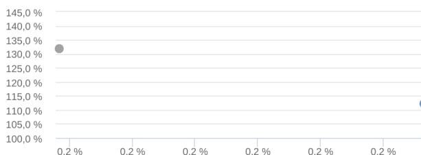
Risco x Retorno - 29/04/2011 a 22/04/2021 (diária)
