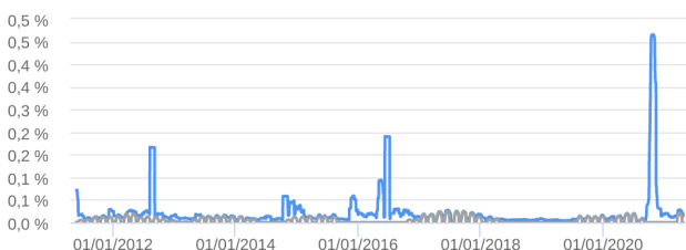
Volatilidade Anualizada - 29/04/2011 a 22/04/2021 (diária)
