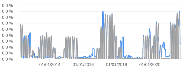
Volatilidade Anualizada - 17/02/2012 a 28/10/2021 (diária)
