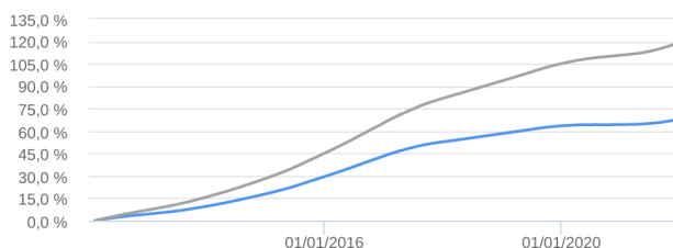
Retorno Acumulado - 17/02/2012 a 27/12/2021 (diária)
