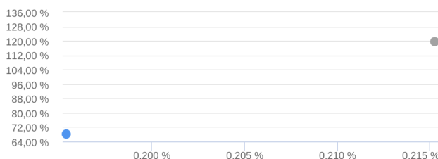
Risco x Retorno - 17/02/2012 a 27/12/2021 (diária)
