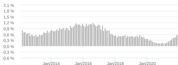
Retorno Mensal - 17/02/2012 a 27/12/2021 (mensal)
