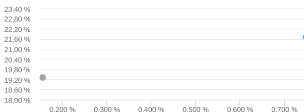
Risco x Retorno - 16/10/2018 a 10/05/2022 (diária)
