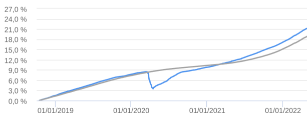
Retorno Acumulado - 16/10/2018 a 10/05/2022 (diária)
